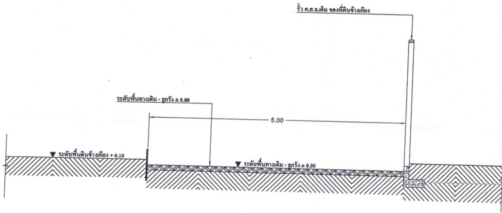
รูปตัด ก - ก (ก่อนดำเนินการ) 1 : 50
