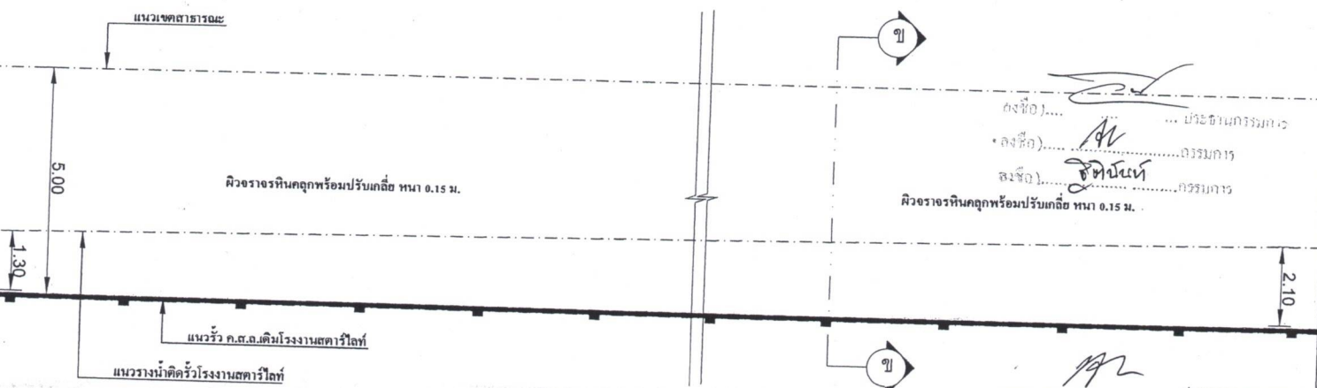
แปลนขยายคูระบายน้ำ (ดำเนินการแล้วเสร็จ กม.0+252.50 - 0+514.10) 1:100
