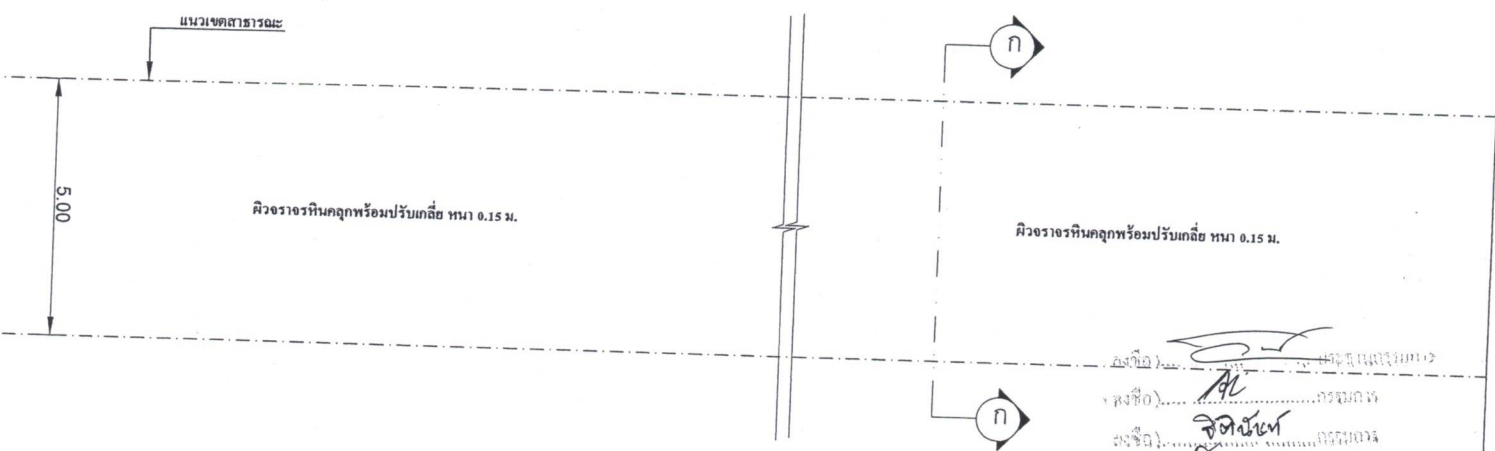
แปลนขยายผิวจราจร (ดำเนินการแล้วเสร็จ กม.0+000.00 - 0+252.50) 1 : 100
