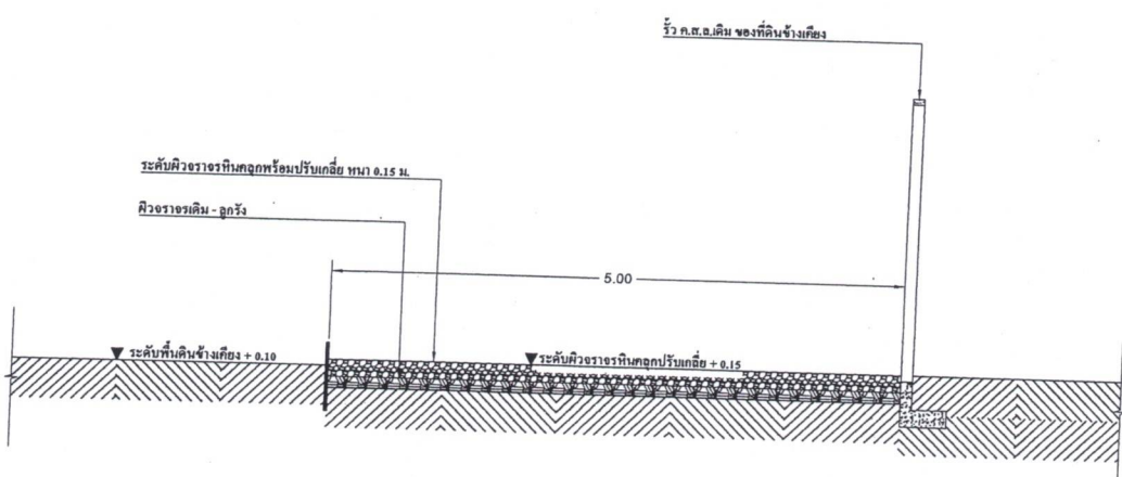
รูปตัด ก - ก (ดำเนินการแล้วเสร็จ) 1 : 50
